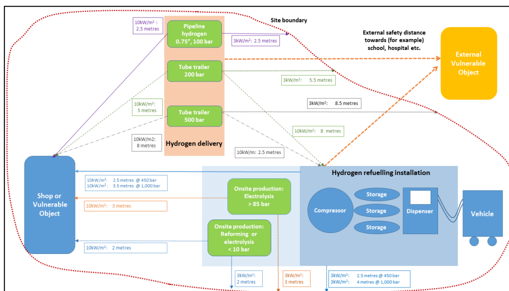
Figuur C.1 — Interne veiligheidsafstanden
